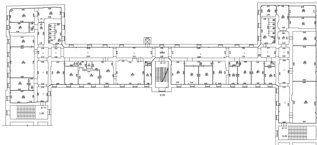
План части 4-го этажа
